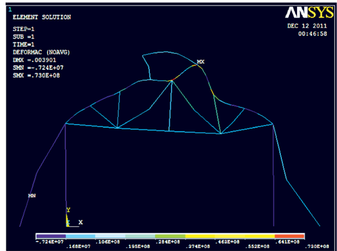
FIGURA 9. Esfuerzos.
