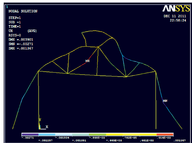
FIGURA 10. Deformaciones.
