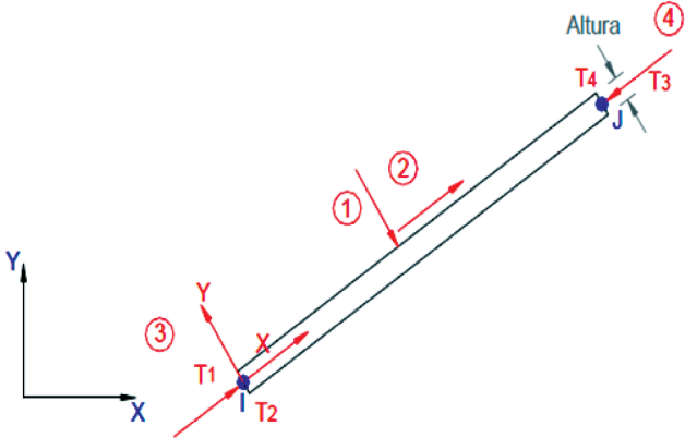
FIGURA 5. Elemento BEAM3.
