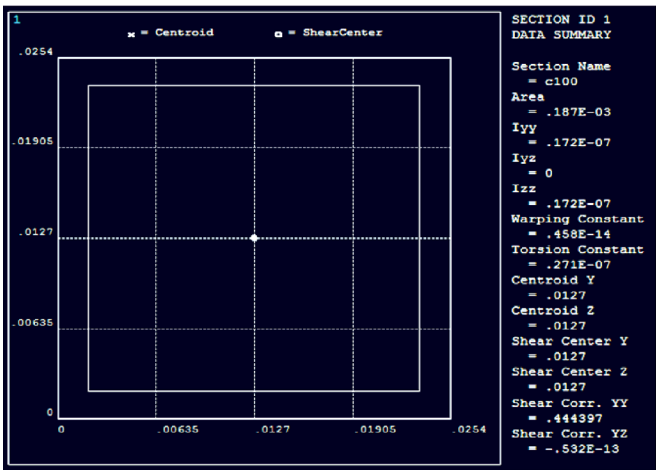
FIGURA 6. Dimensionamiento del elemento BEAM3.
