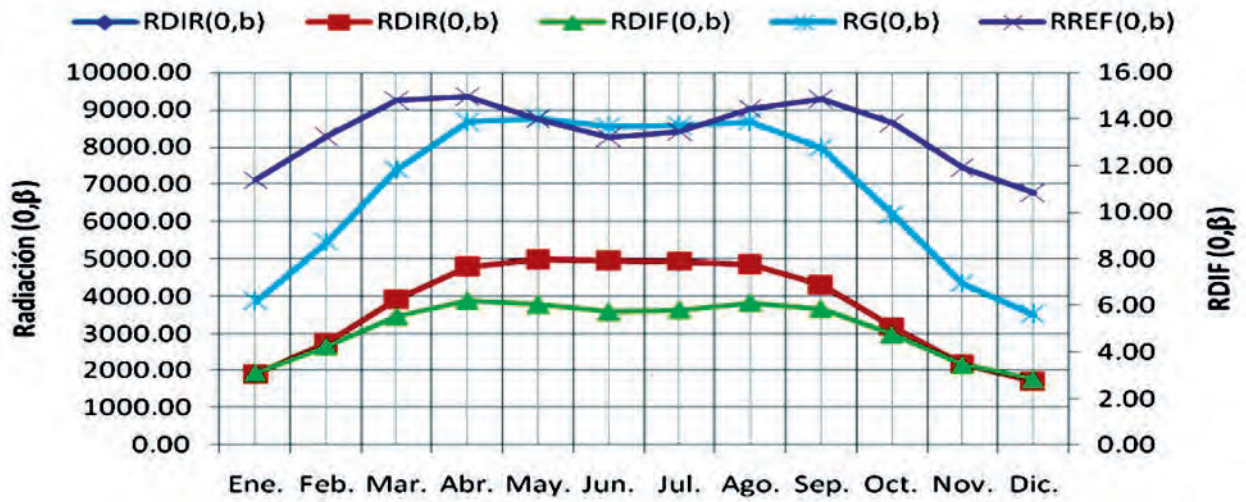
FIGURA 2. Componentes de la radiación con una inclinación de 12.5°.
