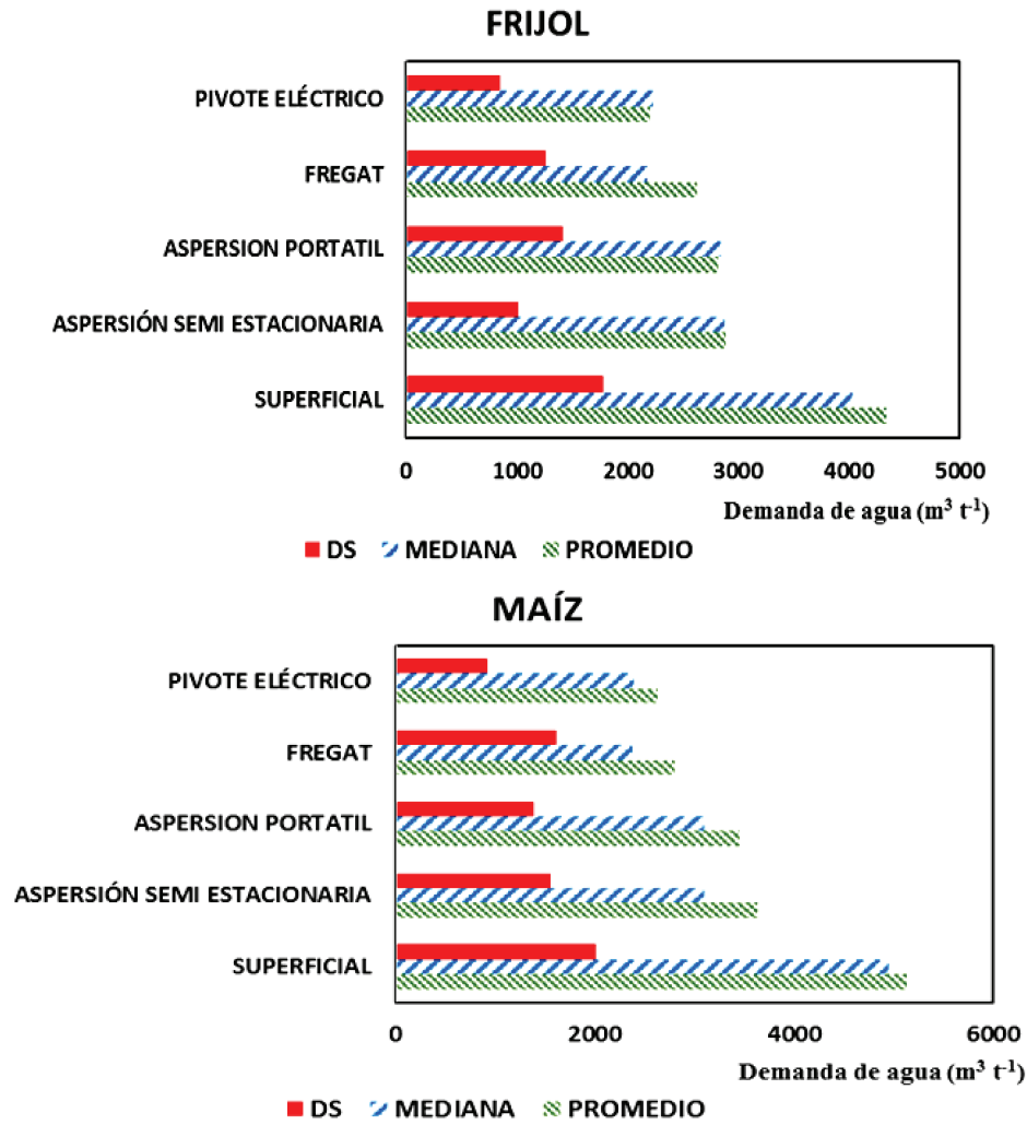
FIGURA 3. Demanda de agua de riego bruta y variabilidad de la demanda (DS) para producir una tonelada de frijol y maíz.
