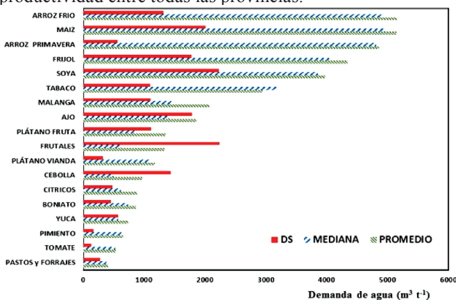
FIGURA 2. Promedio, mediana y desviación estándar de la demanda de agua por tonelada de producción según el cultivo ( \text{m}^3 \text{t}^{-1} ) para el riego superficial.
