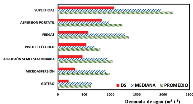
FIGURA 1. Promedio, mediana y desviación estándar de la demanda de agua por tonelada de producción ( \text{m}^3 \text{t}^{-1} ) según la técnica de riego.
