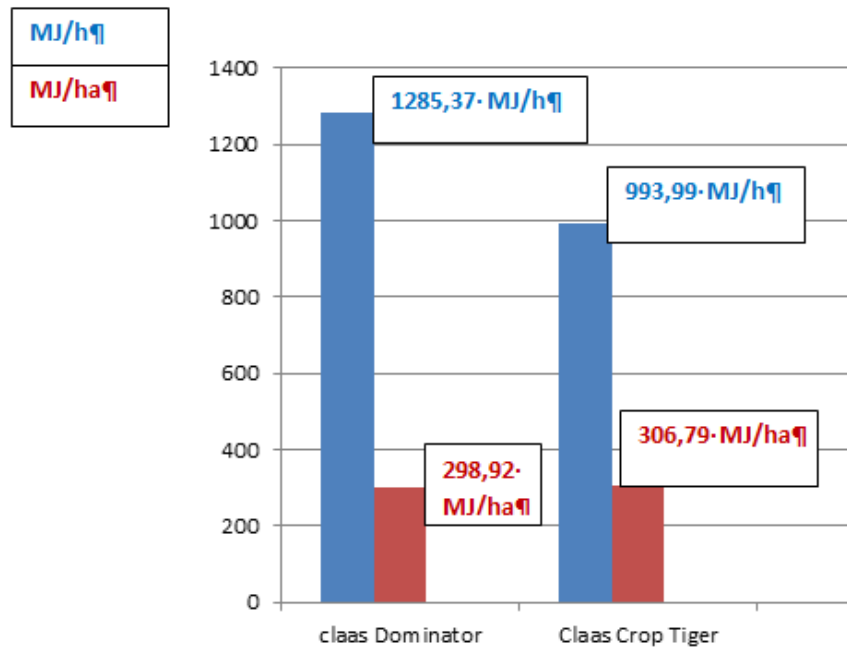
FIGURA 3. Comparación del Costo Energético de las cosechadoras Claas Crop Tiger C-210 y Claas Dominator 130.
