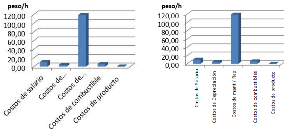
FIGURA 4. Costos de explotación de la cosechadora Claas Crop Tiger C-210.
