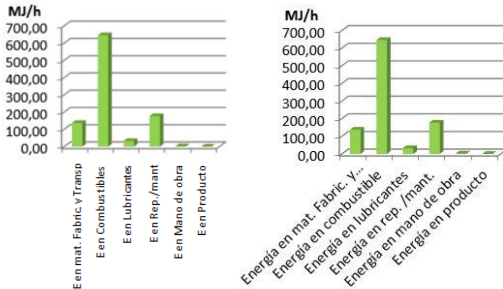
FIGURA 1. Energía requerida de la cosechadora Claas Crop Tiger C-210.
