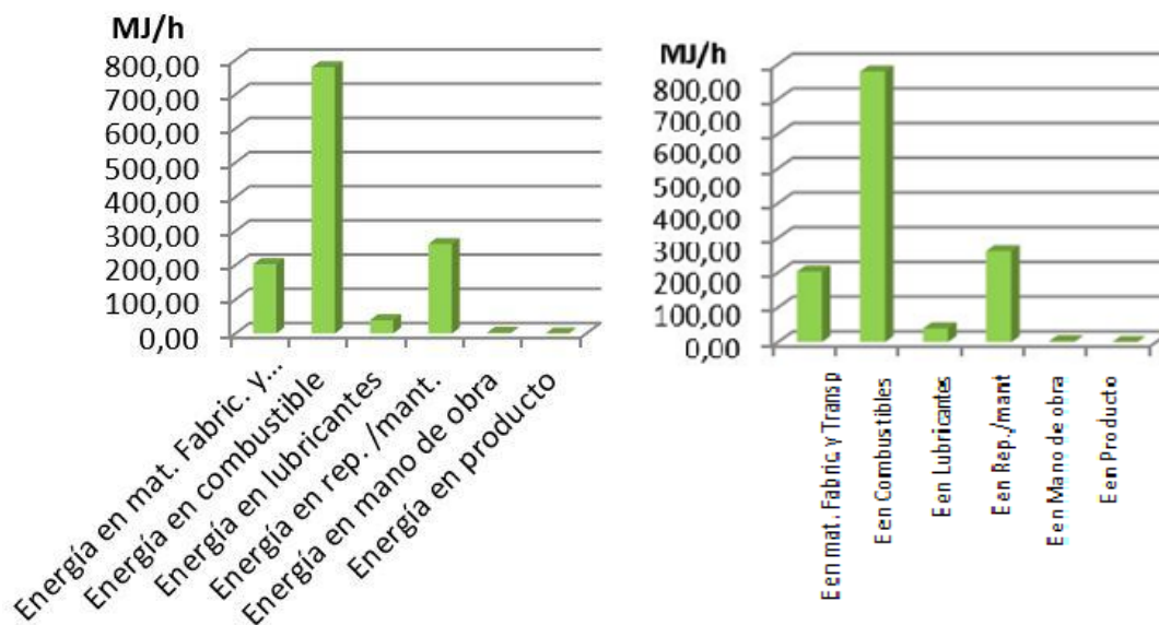
FIGURA 2. Energía requerida de la cosechadora Claas Dominator 130.
