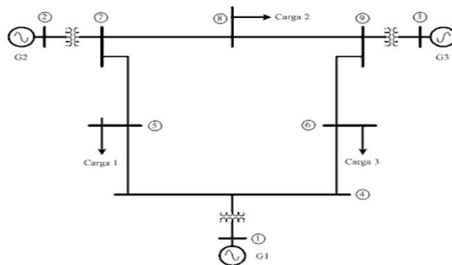
Fig. 3. Sistema típico de 9 barras de la IEEE.
