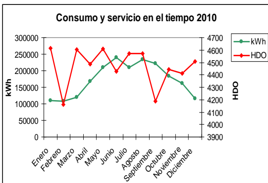
Fig. 5. Consumo (kWh) vs. Nivel ocupacional (HDO), La Pradera 2010.
