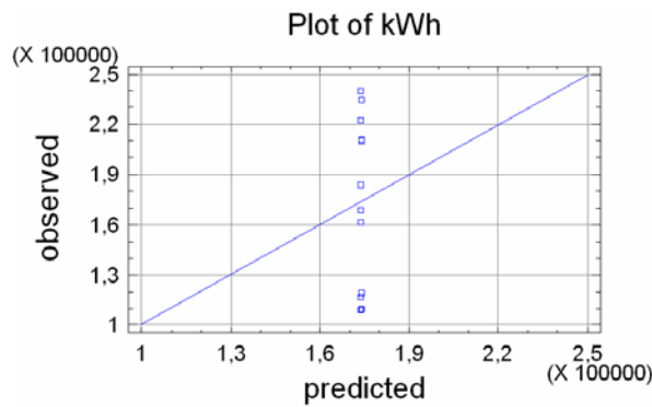
Fig. 9. Comparación de valores de consumo de electricidad observados y predichos por el modelo, La Pradera 2010.
