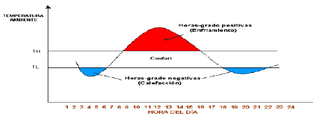
Fig. 2. Visualización gráfica del concepto de horas-grado [10].
