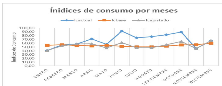
Fig. 7. Comparación gráfica anual entre índices de consumo.
