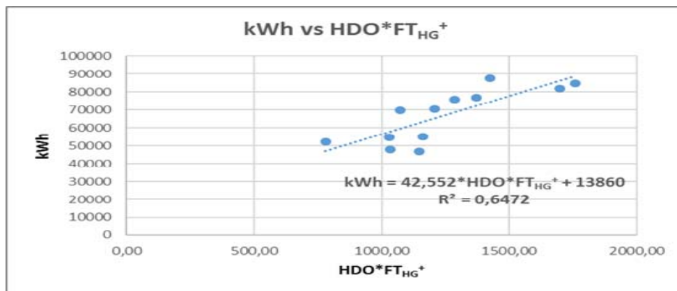
Fig. 6. Relación entre consumo energético (kWh) y la expresión HDO F_{tHG^+} .
