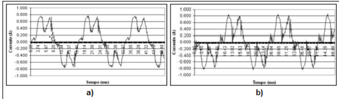
Fig. 5. Forma de onda de corrente de lâmpada a vapor de mercúrio e forma de onda de corrente de lâmpada a vapor de sódio.
