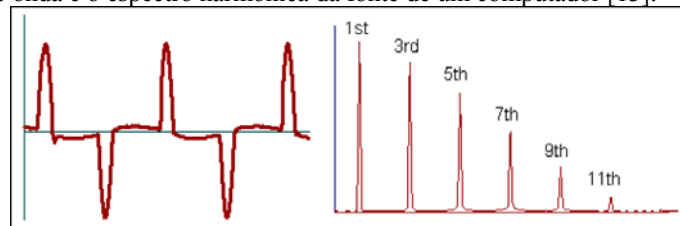
Fig. 7. Forma de onda e o espectro harmónica da fonte dum computador.
