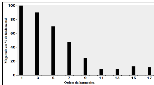
Fig. 6. Espectro harmónica de uma lâmpada a vapor de sódio e a vapor de mercúrio. Computadores.
