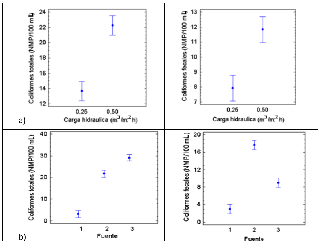
Figura 2. Concentración de coliformes fecales y totales en el efluente de los bioreactores: a) carga hidráulica; b) tipos de fuentes: (1) Cascada Juan González, (2) río Carpintero, (3) finca Porvenir
