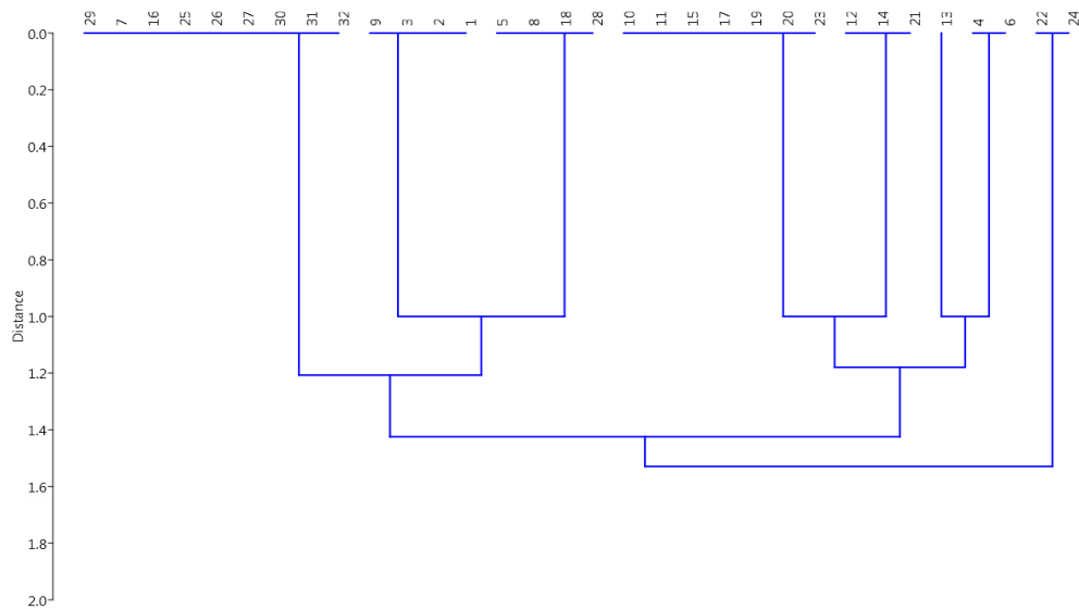
Figura 2. Dendrograma de convergencia
