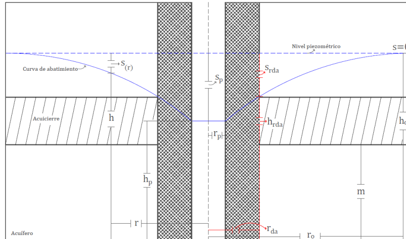
Fig. 1. - Imagen general de un pozo sin camisa y filtro artificial de grava en un acuífero confinado, considerando las actividades de desarrollo.
