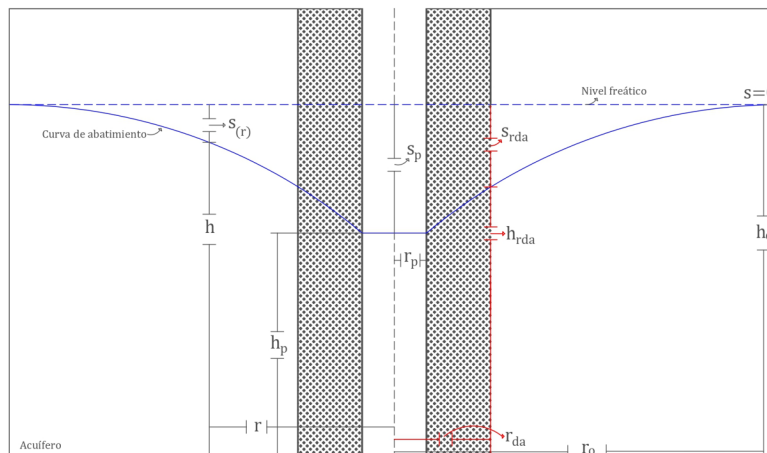
Fig.2. - Imagen general de un pozo sin camisa y filtro artificial de grava en un acuífero libre, considerando las actividades de desarrollo.
