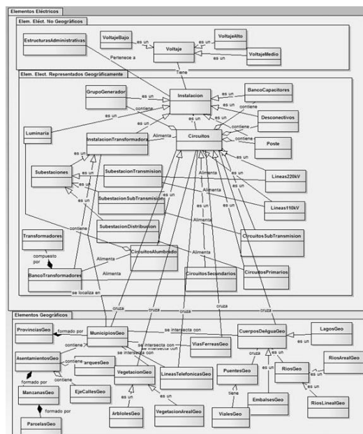
Fig. 3. Diagrama de clases de los elementos eléctricos básicos según su representación geográfica
