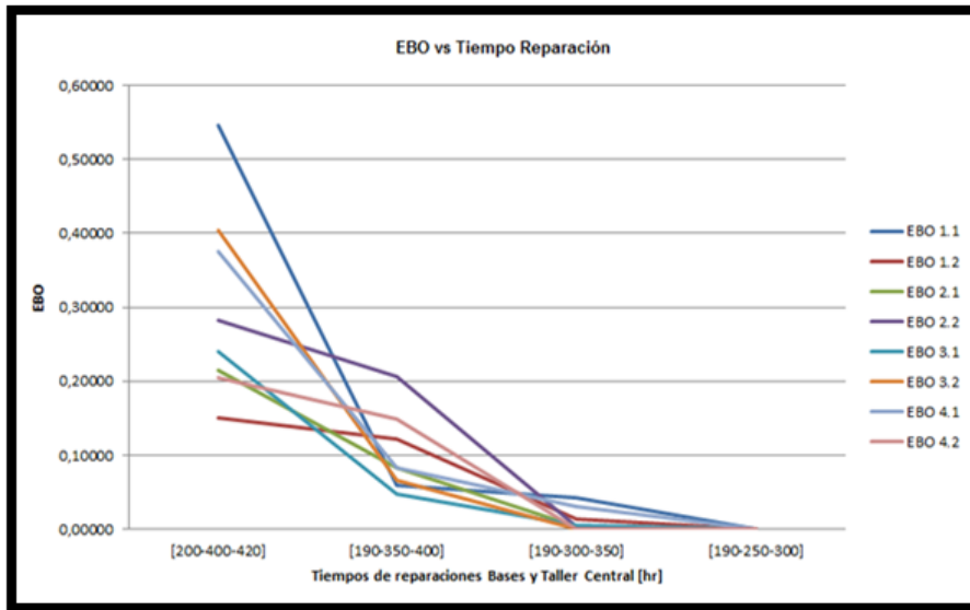
Fig. 8. Variación valores de EBO para cada elemento en su lugar respectivo
