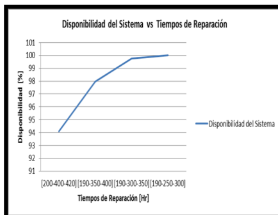
Fig. 9. Disponibilidad del sistema en función de los tiempos de reparación de las bases y taller central
