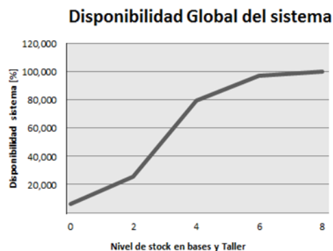
Fig. 3. Disponibilidad del Sistema vs. Niveles de stock
