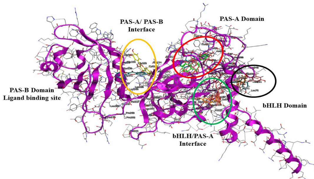
Figura 4. Flavonoides activos que interfieren las IPP de AHR con ARNT a nivel dominio bHLH de AHR. Interfaces bHLH/bHLH (círculo negro), bHLH-PAS-A (círculo verde), PAS-A/PAS-A (círculo rojo) y PAS-A/PAS-B (círculo amarillo).
