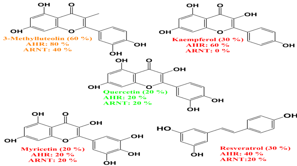
Fig. 3. Estructuras de los cinco flavonoides moduladores de la actividad de AHR. Porcentajes de interferencia de la formación del heterodímero funcional AHR: ARNT y a nivel de los monómeros AHR y ARNT.
