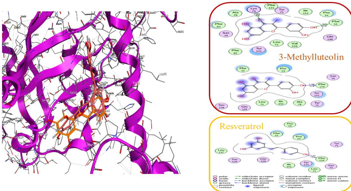
Fig. 6. Flavonoides activos que interfieren las IPP de AHR con ARNT a nivel de la interface bHLH/PAS-A de AHR. Methylluteolin (rosado), Resveratrol (anaranjado). AHR (magenta).
