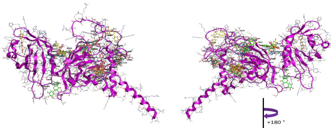
Fig. 2. Representación esquemática de la unión de cinco flavonoides en AHR (AHR SwissModel). Color magenta.
