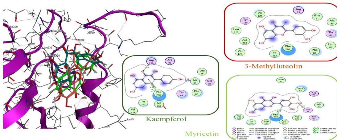
Fig. 7. Flavonoides activos que interfieren las IPP de AHR con ARNT a nivel de la interfase PAS-A de AHR. Methyluteolin (rosado), Kaempferol (verde olivo), Myricetin (verde). AHR (magenta).
