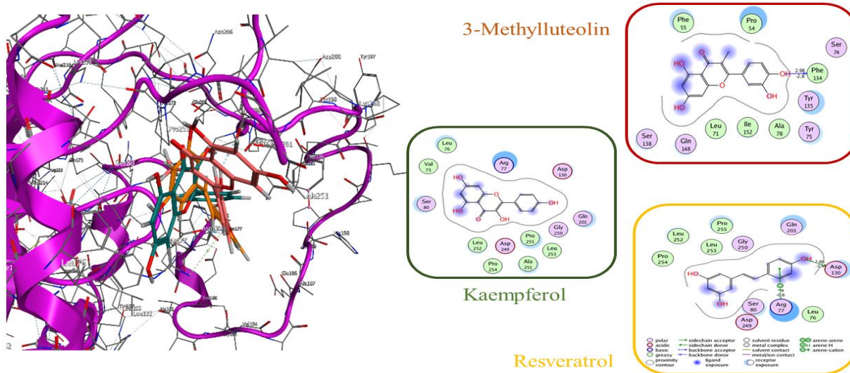
Fig. 5. Flavonoides activos que interfieren las IPP de AHR con ARNT a nivel dominio bHLH/bHLH de AHR. Methylluteolin (rosado), Kaempferol (verde olivo), Resveratrol (anaranjado). AHR (magenta).
