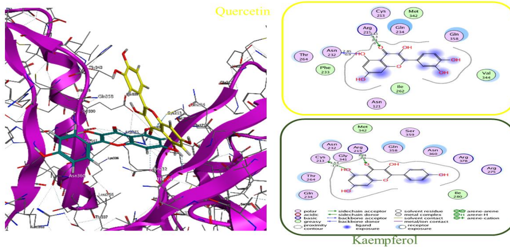
Fig. 8. Flavonoides activos que interfieren las IPP de AHR con ARNT a nivel de la interface PAS-A/PAS-B de AHR. Quercetin (amarillo), Kaempferol (verde olivo), Myricetin (verde). AHR (magenta).
