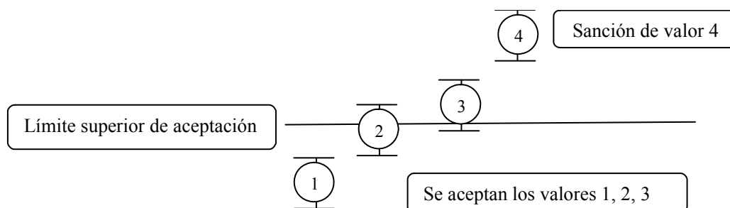
FIGURA. Intervalos de los valores y la incertidumbre expandida en relación con el límite de aceptación./ Value intervals and the expanded uncertainty in relation to the acceptance limit.
