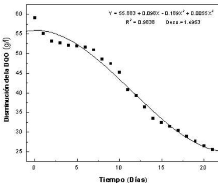
Fig. 4 Cambio de la demanda química de oxígeno a través del tiempo.
