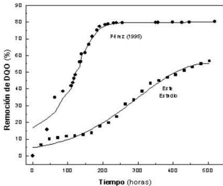
Fig. 8 Comparación del porcentaje de remoción de la DQO.
