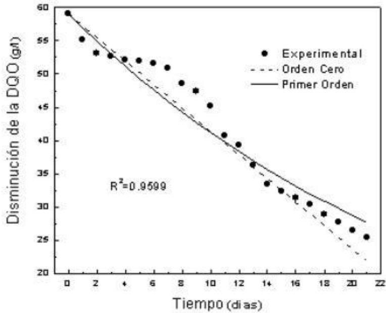
Fig. 7 Representación del orden cinético de la reacción.
