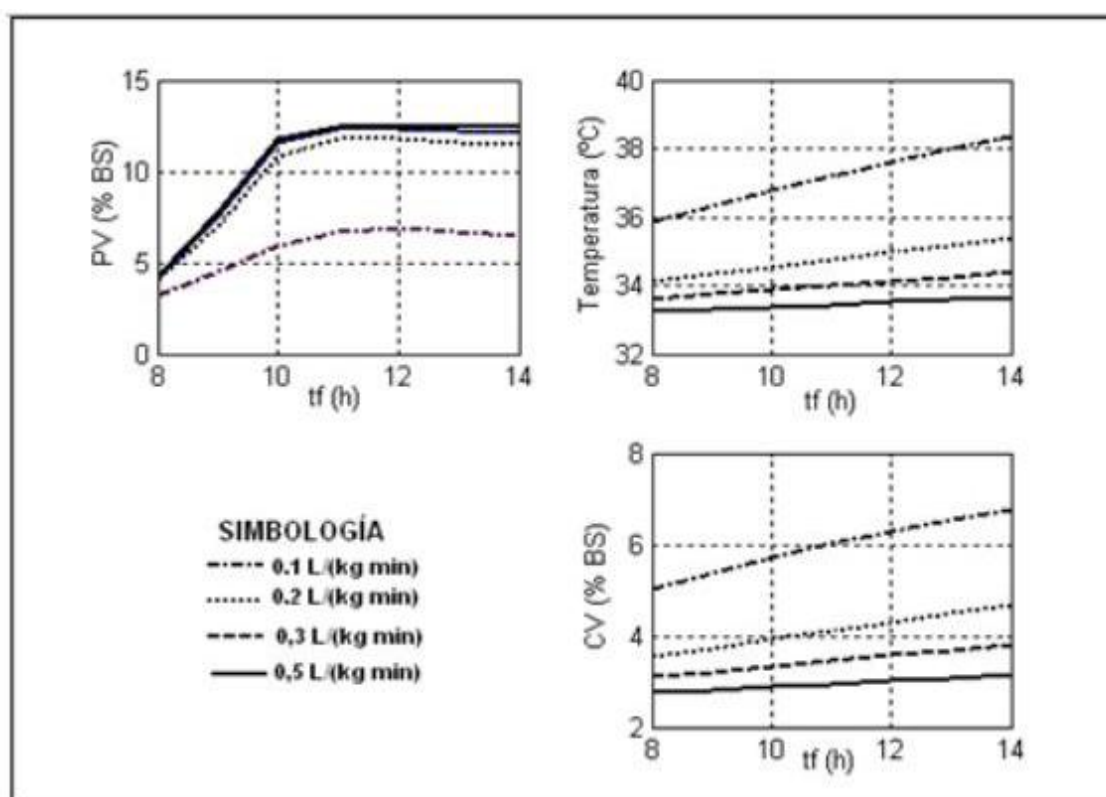
Fig. Sensibilidad del sistema ante las variaciones de tiempo de residencia y flujo específico de aire.
