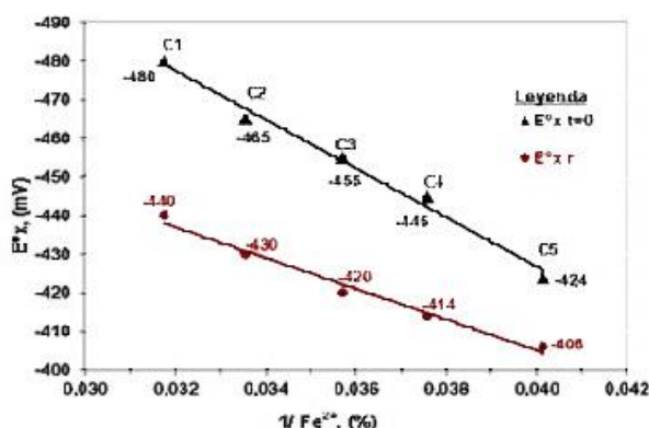
Fig. 2 Interacción entre el potencial redox y el % de Fe 2+ en MR.
