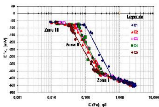
Fig. 1 Comportamiento del Potencial Redox y Ci de MR.
