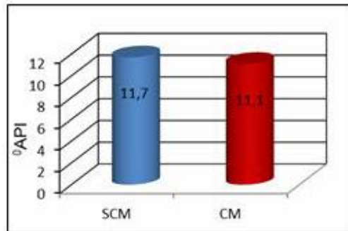
Fig.6 Gravedad API determinada para el crudo PCNm-1400 sin tratar y tratado magnéticamente
