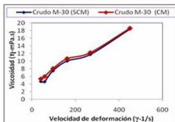
Fig.1 Efecto del tratamiento magnético en la viscosidad del crudo M-30
