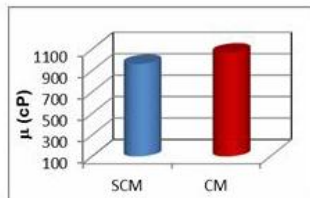
Fig.7 Viscosidad cinemática determinada para el crudo PCNm-1400 sin tratar y tratado magnéticamente
