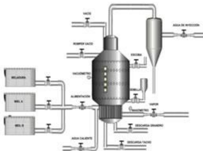
Figura 2. Esquema funcional del tacho cristalizador
