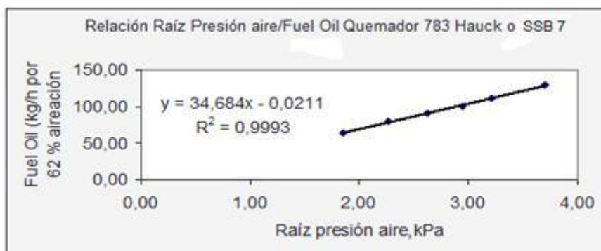
Fig. 4 Relación Fuel oil vs Presión de aire del quemador 783 Hauck o PriorSSB 7.
