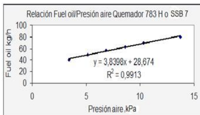
Fig. 2 Relación Fuel oil vs Presión de aire del quemador 783 Haucko PriorSSB 7.
