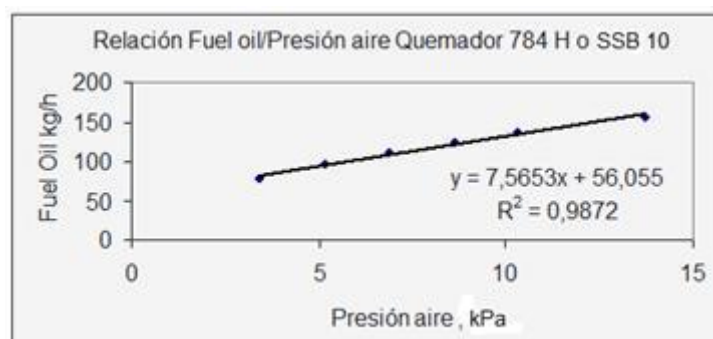
Fig. 3 Relación Fuel oil vs Presión de aire del quemador 784 Haucko PriorSSB 10.
