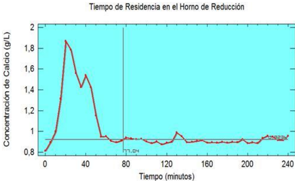
Fig. 2 Comportamiento de la concentración de calcio dentro del horno de solera múltiple.
