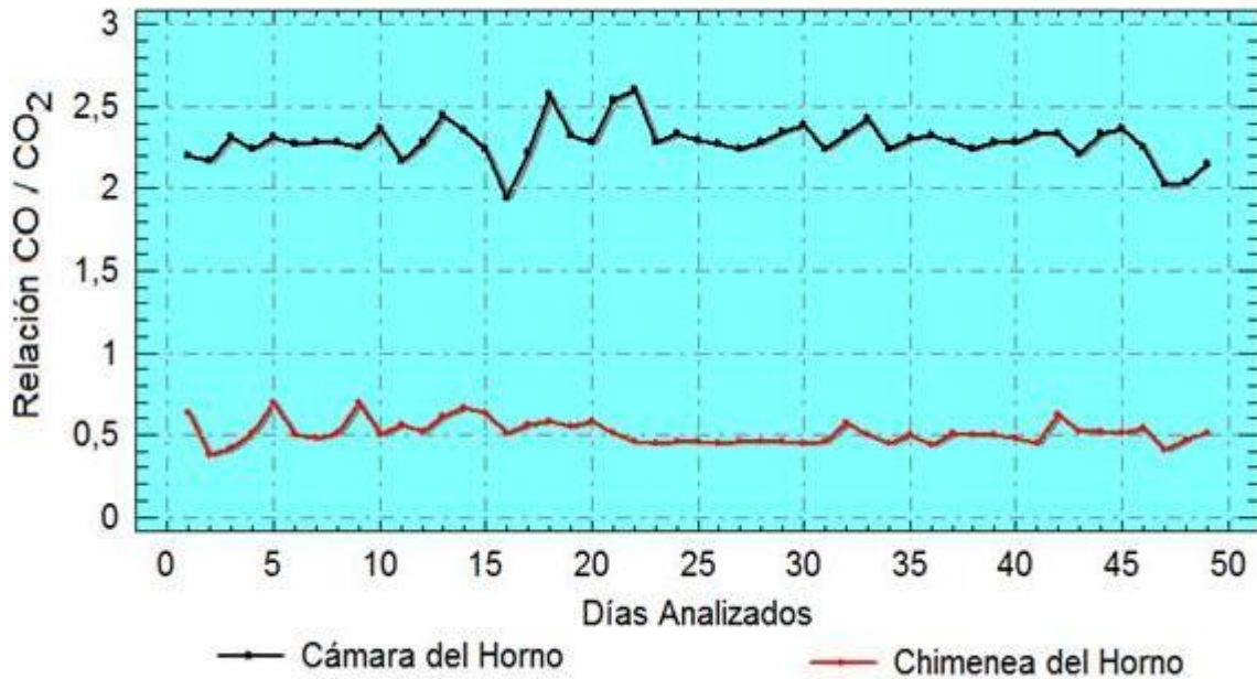
Fig. 5 Relación volumétrica entre el CO y el CO 2 en el horno a escala piloto.
