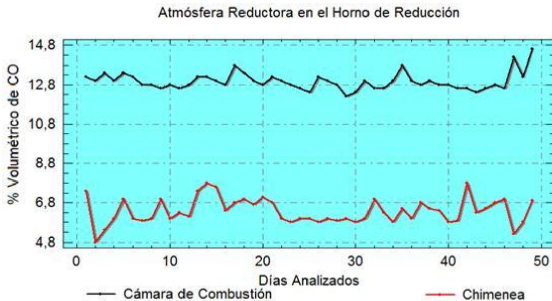
Fig. 6 Relación volumétrica del CO en el horno.
