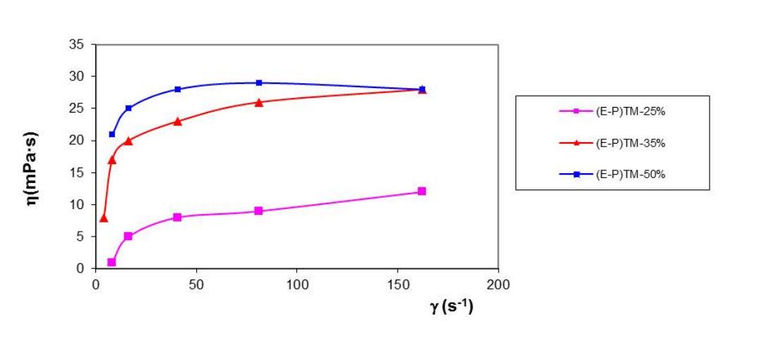
Fig. 5 Viscosidad de emulsiones tratadas magnéticamente con emulgente P,
