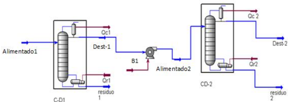
Fig. N° 1. Diagrama de flujo obtenido con el simulador HYSYS para la situación problémica 1
