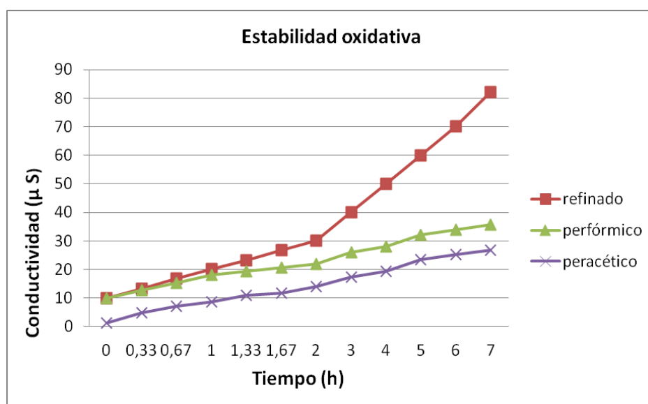
Figura 2. Resultados del ensayo Rancimat del aceite refinado de Jatropha curcas L. y de los productos epoxidados.
