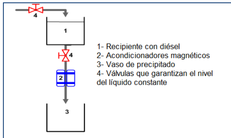
Figura 3. Esquema del tratamiento magnético del combustible.
