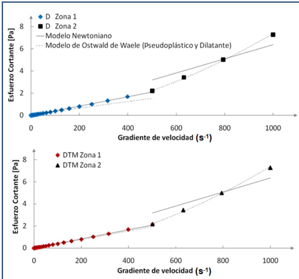
Figura 6. Curvas de flujo de las muestras de diésel sin tratamiento magnético (D) y de diésel tratado magnéticamente (DTM), analizadas por zonas.
