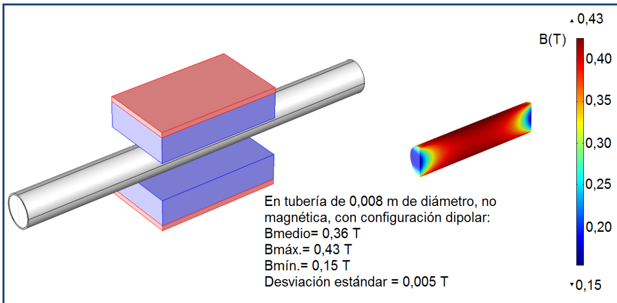
Figura 2. Patrón de distribución de campo magnético en una tubería diamagnética ( B - inducción magnética, B_{\text{máx.}} - inducción máxima, B_{\text{mín.}} - inducción mínima).
