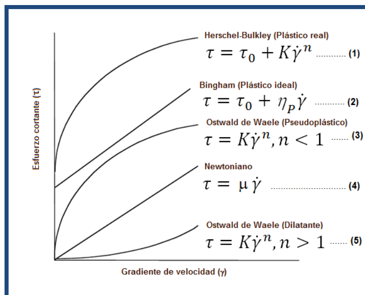
Figura 1. Modelos reológicos independientes del tiempo. [16; 17]
