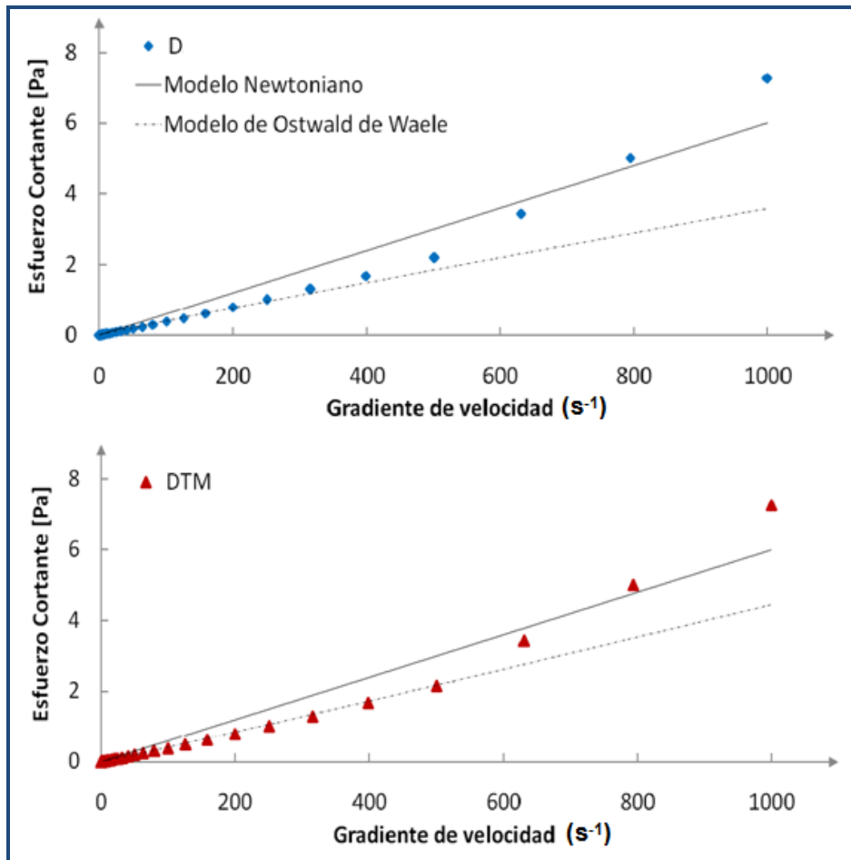
Figura 5. Curvas de flujo de las muestras de diésel sin tratamiento magnético (D) y de diésel tratado magnéticamente (DTM).
