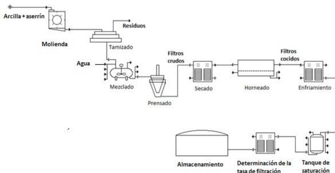
Fig. 1 Diagrama de flujo de la producción del filtro de cerámica “tradifiltro” para la purificación de agua.
