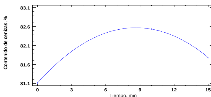
Fig. 4 Curva obtenida del contenido de cenizas a diferentes tiempos.
