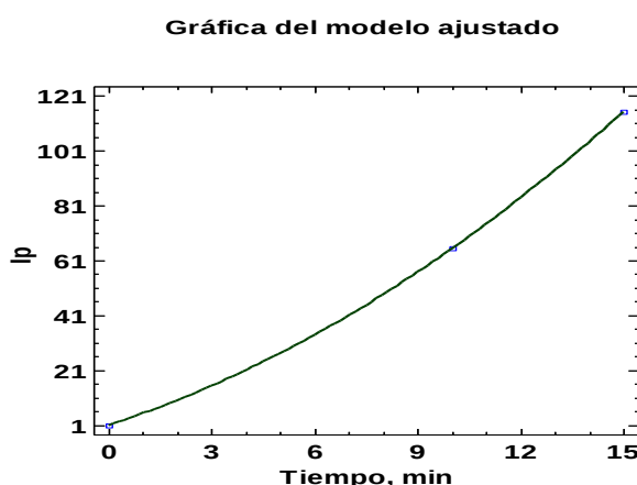
Fig. 5 Índice de mezcla conseguido para la pasta de arcilla y aserrín obtenida en el mezclador.
