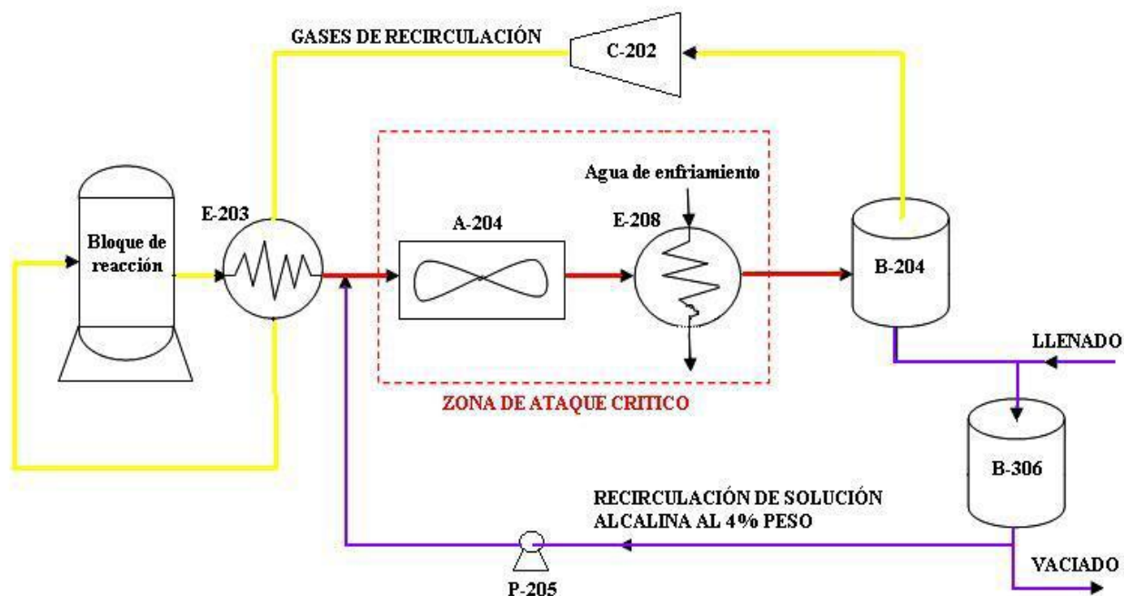
Figura 1. Esquema simplificado de la planta de reformación catalítica.
