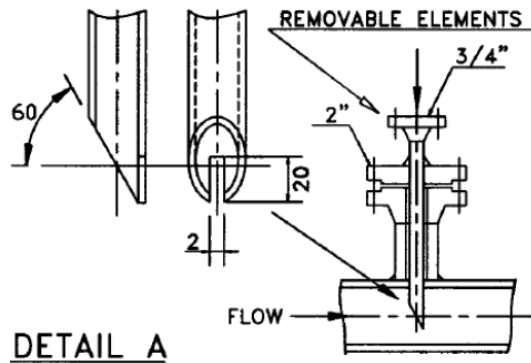
Figura 3. Sistema de inyección de álcali empleado.
