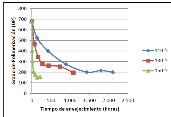
Fig. 2. Grado de Polimerización para diferentes temperaturas de funcionamiento
