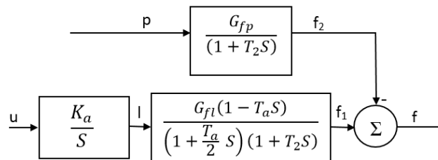
Fig. 5- Diagrama de bloques del modelo de una micro-hidroeléctrica. Fuente (Domínguez, 1999)
