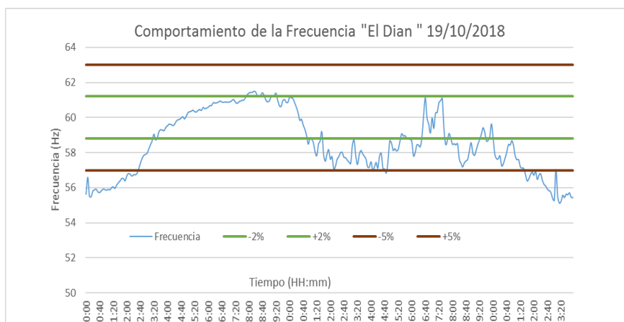
Fig. 3- Comportamiento típico de la Frecuencia de una micro-Hidroeléctrica sin regulación.
