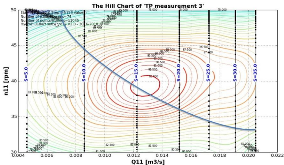
Fig. 2- Curva característica de trabajo de turbinas hidráulicas. Fuente: adaptado de HydroHillChart (15)
