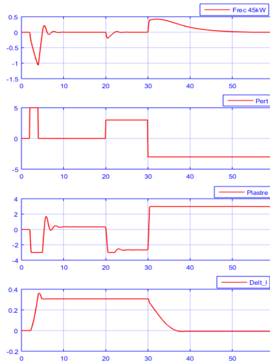
Fig.7- Respuesta de la planta con los métodos de regulación combinada ante perturbaciones de carga en el rango de la potencia secundaria. Fuente: (Autores, 2019).
