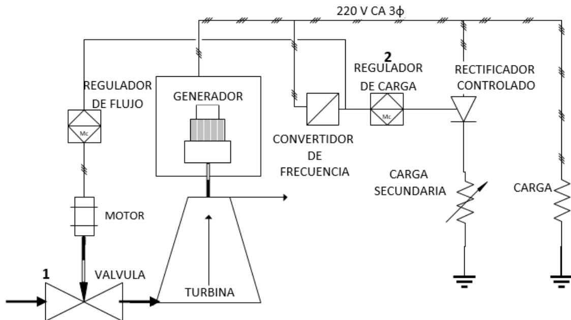
Fig. 4- Esquema de regulación combinado de micro-hidroeléctricas autónomas. 1) Regulación por flujo, 2) Regulación por carga. Fuente: (Autores, 2019)
