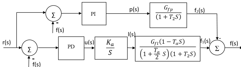
Fig. 6- Diagrama de bloques del sistema de control combinado. Fuente: (Autores, 2019)
