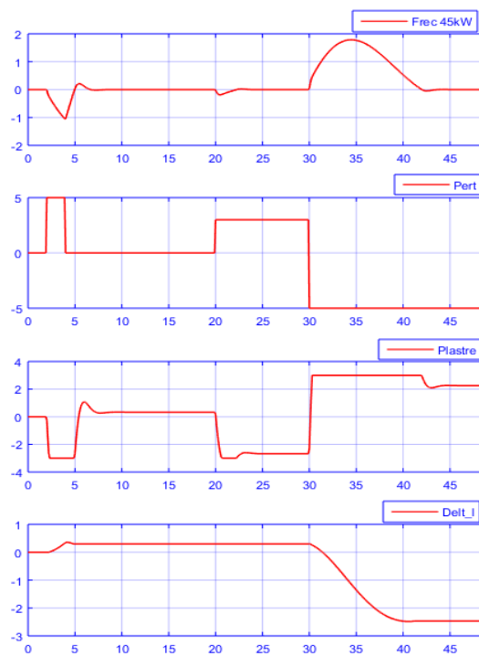
Fig. 8. Respuesta la planta con los métodos de regulación combinada ante perturbaciones mayores que la potencia secundaria. Fuente: (Autores, 2019).
