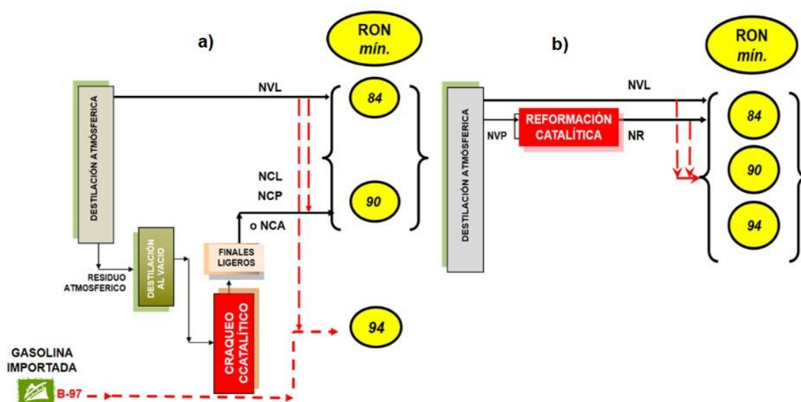
Fig.3- Tecnologías de producción nacional de gasolinas:
