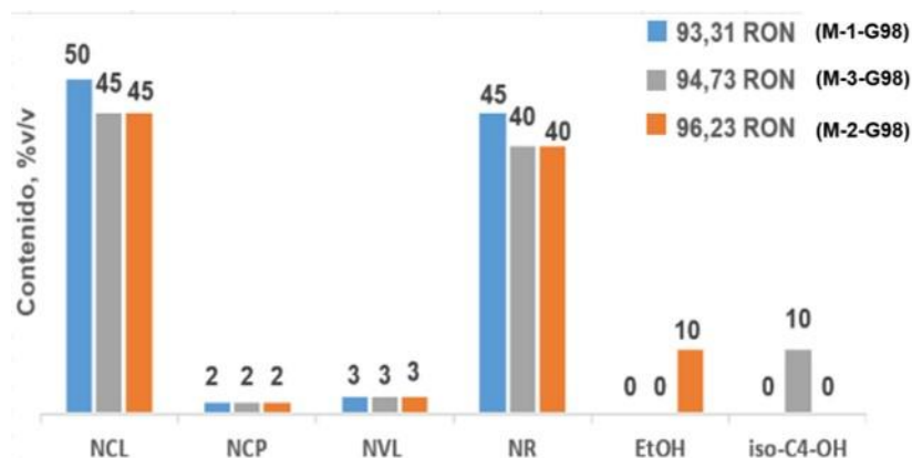
Fig.5- Efecto de alcoholes sobre RON de mezcla base de naftas
