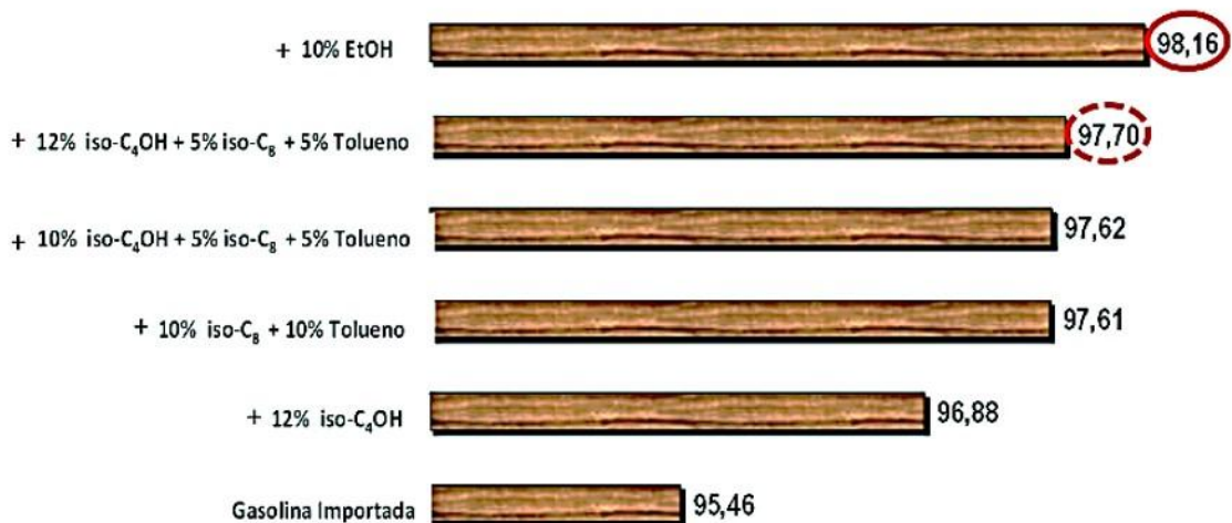
Fig.8- Efecto de componentes mejoradores de octano en el RON de la GI
