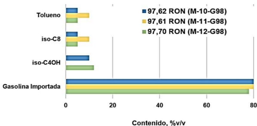
Fig.9- Influencia de alcoholes e hidrocarburos puros en el octano de la GI
