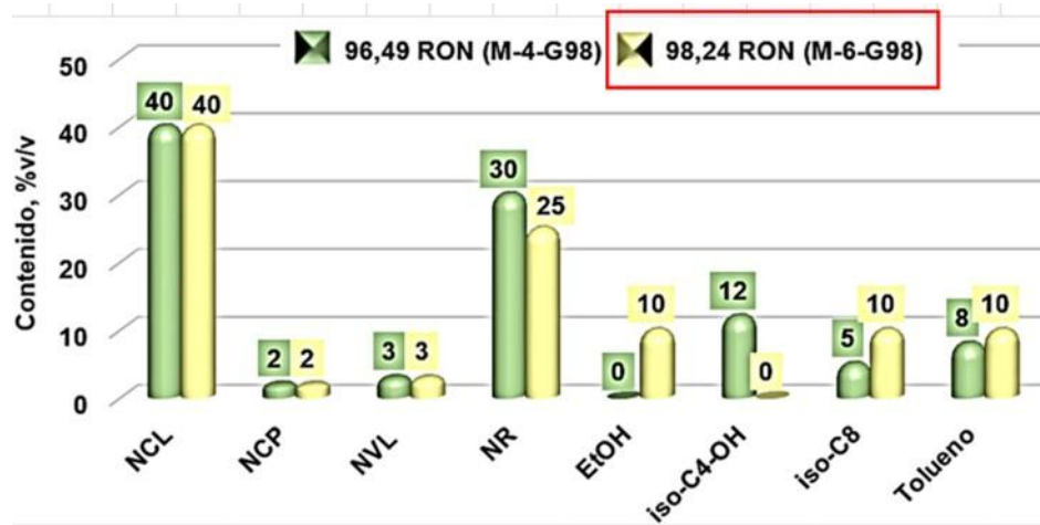
Fig.7- Efecto combinado de alcoholes e hidrocarburos puros
