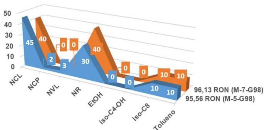
Fig.6- Influencia de la composición hidrocarbonada en RON de mezclas base
