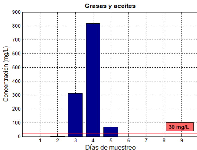
Fig. 2- Comportamiento de las grasas y aceites provenientes del residual.
