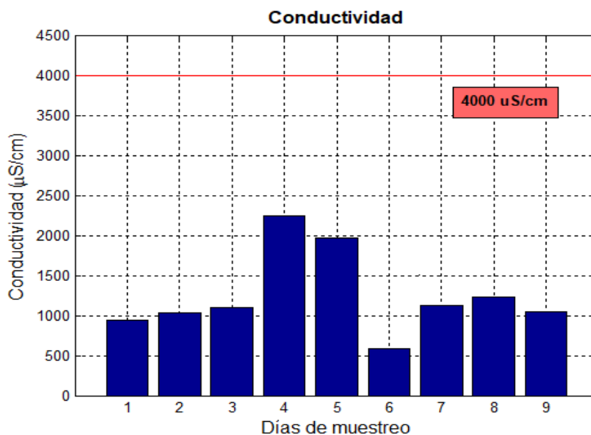
Fig. 3- Comportamiento de la conductividad en el residual.
