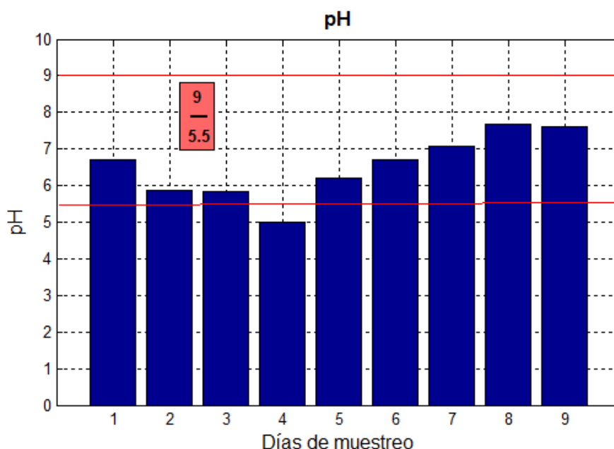
Fig. 4- Comportamiento de los valores del pH en el residual
