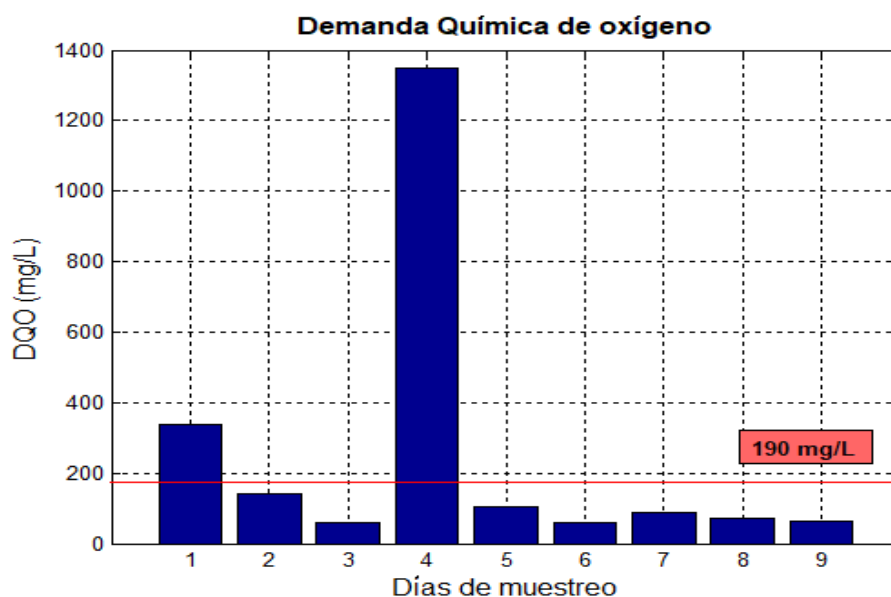
Fig. 5- Comportamiento de la DQO en el residual
