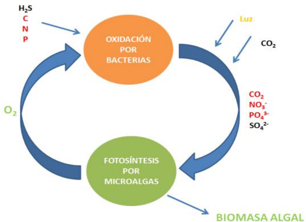
Fig. 1- Interacción simbiótica microalgas - bacterias para la purificación de biogás y tratamiento de aguas residuales simultáneamente; Negro: Purificación de biogás. Rojo: Tratamiento de aguas residuales. Verde: Productos de la fotosíntesis. Fuente: (18)
