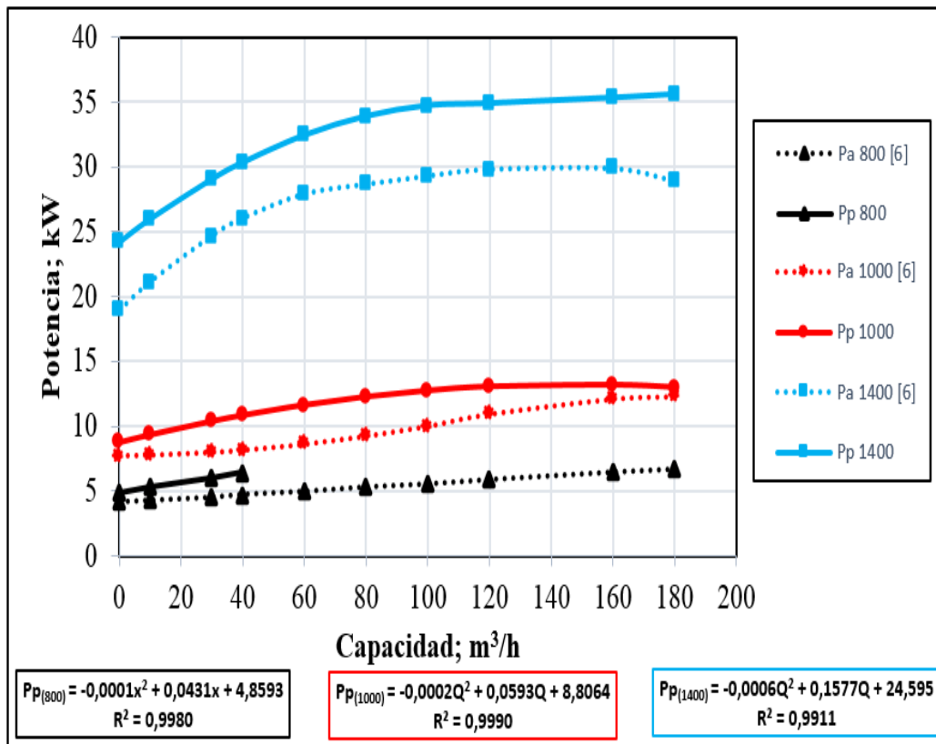
Fig. 2- Curvas características de potencia–capacidad de la bomba centrífuga лG
