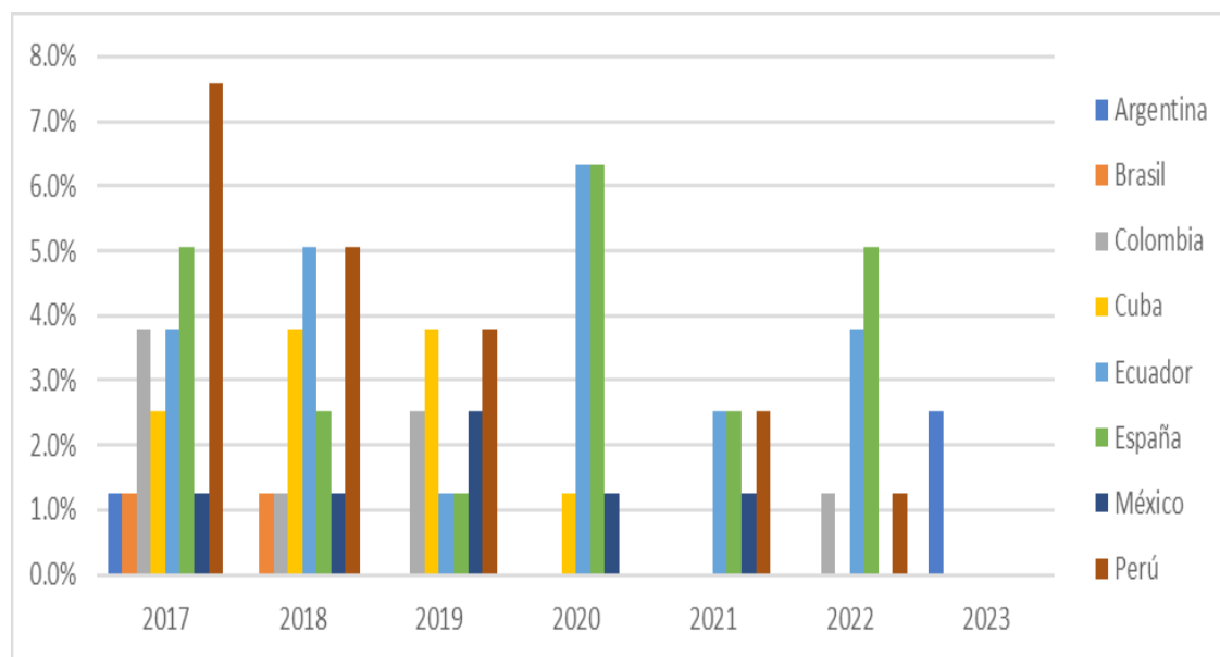
Figura 2: Producción científica según publicaciones por países y años.
