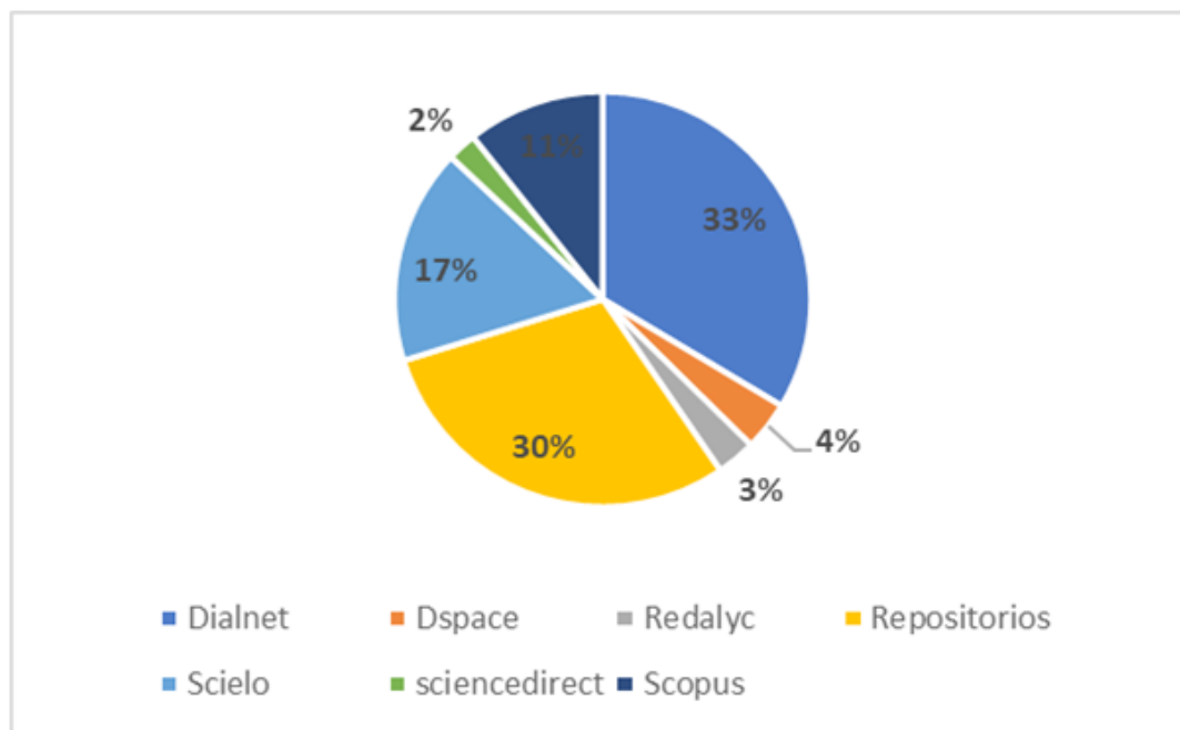
Figura 5: Distribución de los registros informacionales por fuentes de información. Fuente: elaboración propia.
