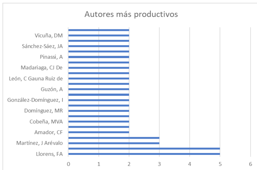
Figura 9: Autores líderes teniendo en cuenta número de publicaciones.
