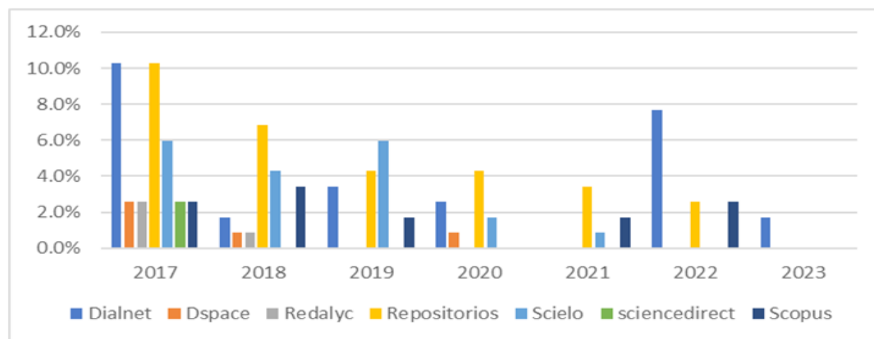
Figura 8: Productividad científica teniendo en cuenta fuentes por años.
