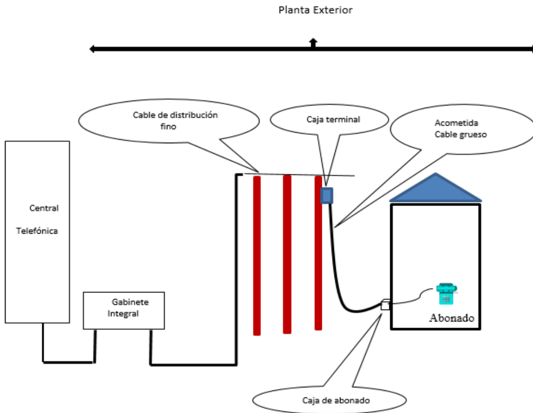
Fig. 1: Elementos de la planta exterior telefónica.
